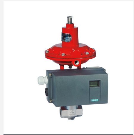
SIPART PS 2 (Siemens)
